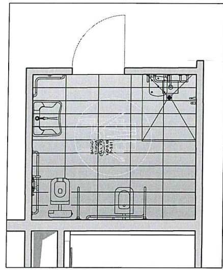
BAGNO DISABILE - STANZE DI DEGENZA
